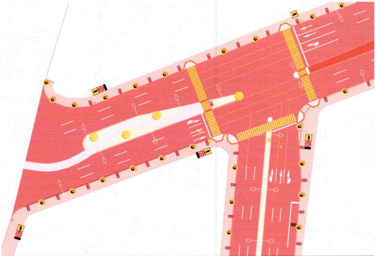
Imagen proyecto propuesta estación de transferencia Metro-Camión Calle Munich
