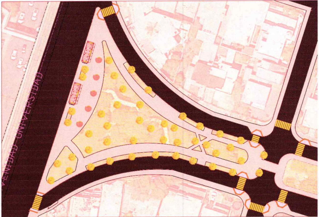
Imagen proyecto geométrico Sor Juana Inés de la Cruz
